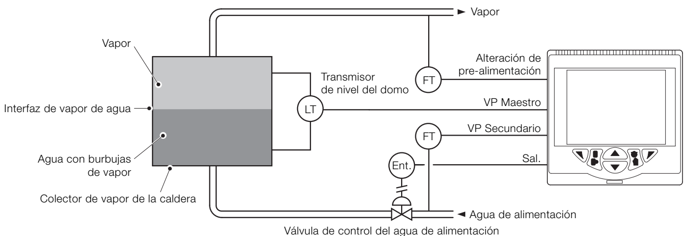
Fig. 22: Cascada con pre-alimentación
