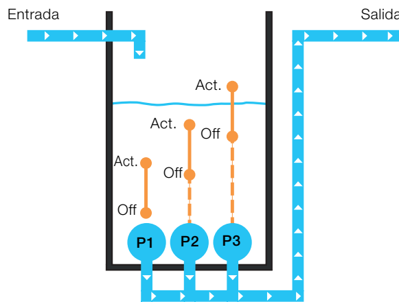
Fig. 13: Puntos de activación y desactivación independientes
