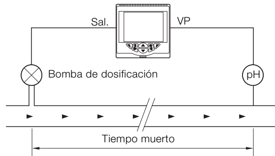
Fig. 8: Ejemplo de control predictivo
