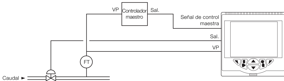
Fig. 25: Estación automática/manual y estación de soporte analógica
