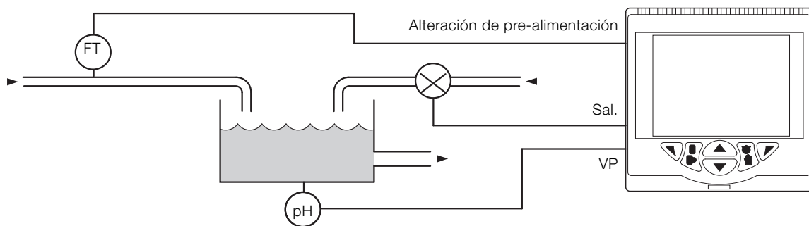
Fig. 20: Lazo simple con pre-alimentación
