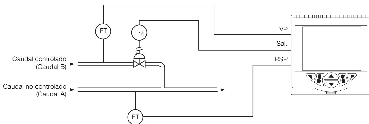
Fig. 23: Controlador de relación
