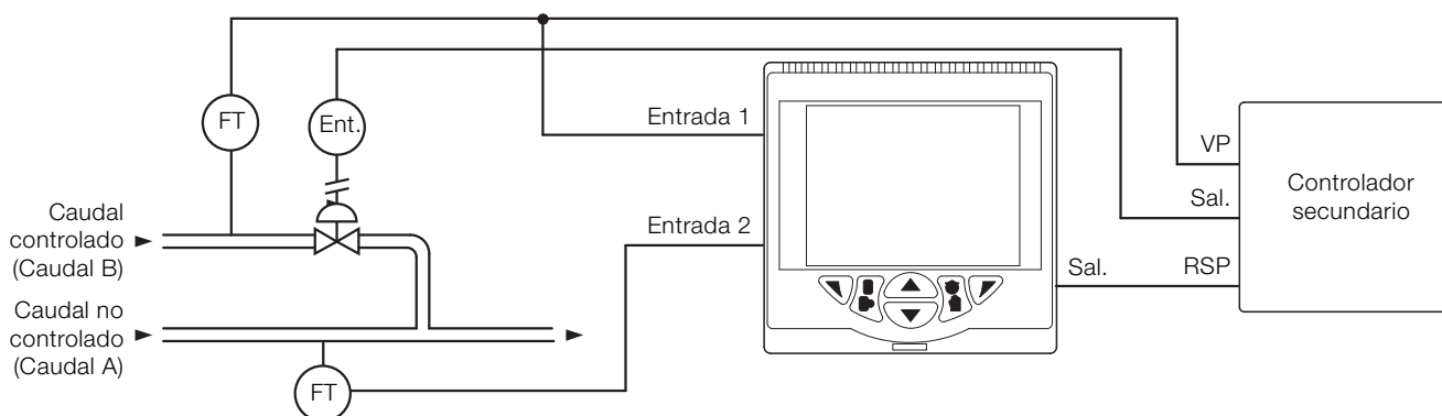
Fig. 24: Estación de relación
