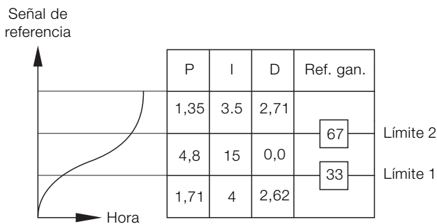
Fig. 7: Ejemplo de programación de la ganancia
