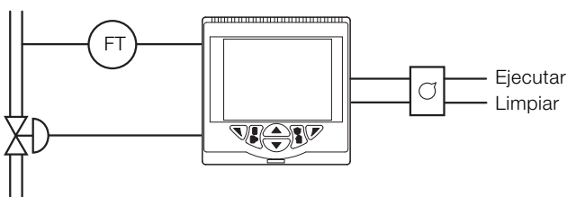
Fig. 11: Conmutación remota automática/manual
