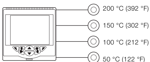
Fig. 12: Selección del punto de consigna externo
