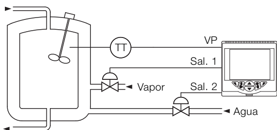
Fig. 10: Ejemplo de control de salida dividida
